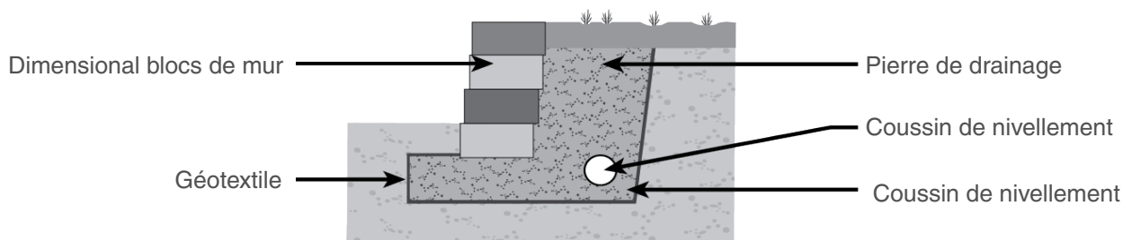
DE SOUTÈNEMENT
